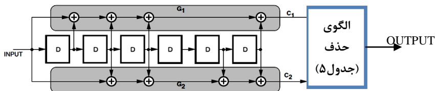
شکل (۳) بلوک دیاگرام کدگذار حذفی (CCSDS 101.0-B-4, 1999)
