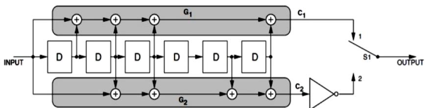
شکل (۲) بلوک دیاگرام کدگذار کانولوشن (CCSDS 101.0-B-4, 1999)
