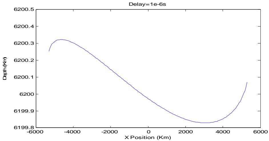
شکل ۹: فاصله از مرکز زمین بر حسب موقعیت X.
